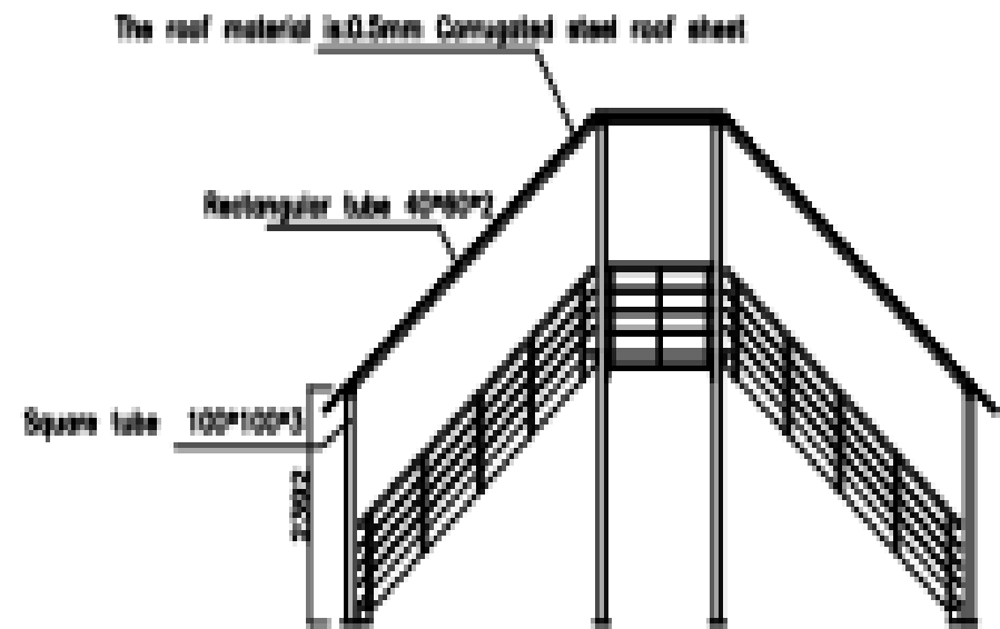
樓梯
